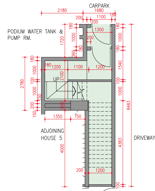
B1/F Floor Plan 地庫一樓樓面平面圖
